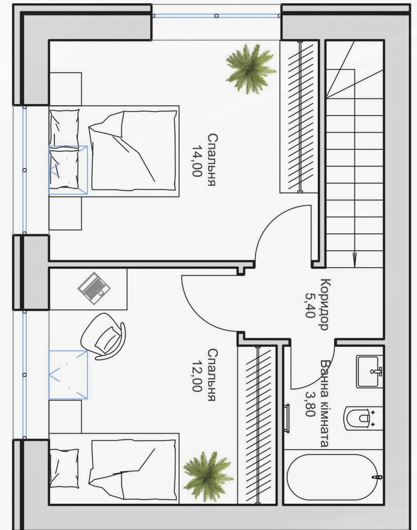
Планування 2-го поверху
