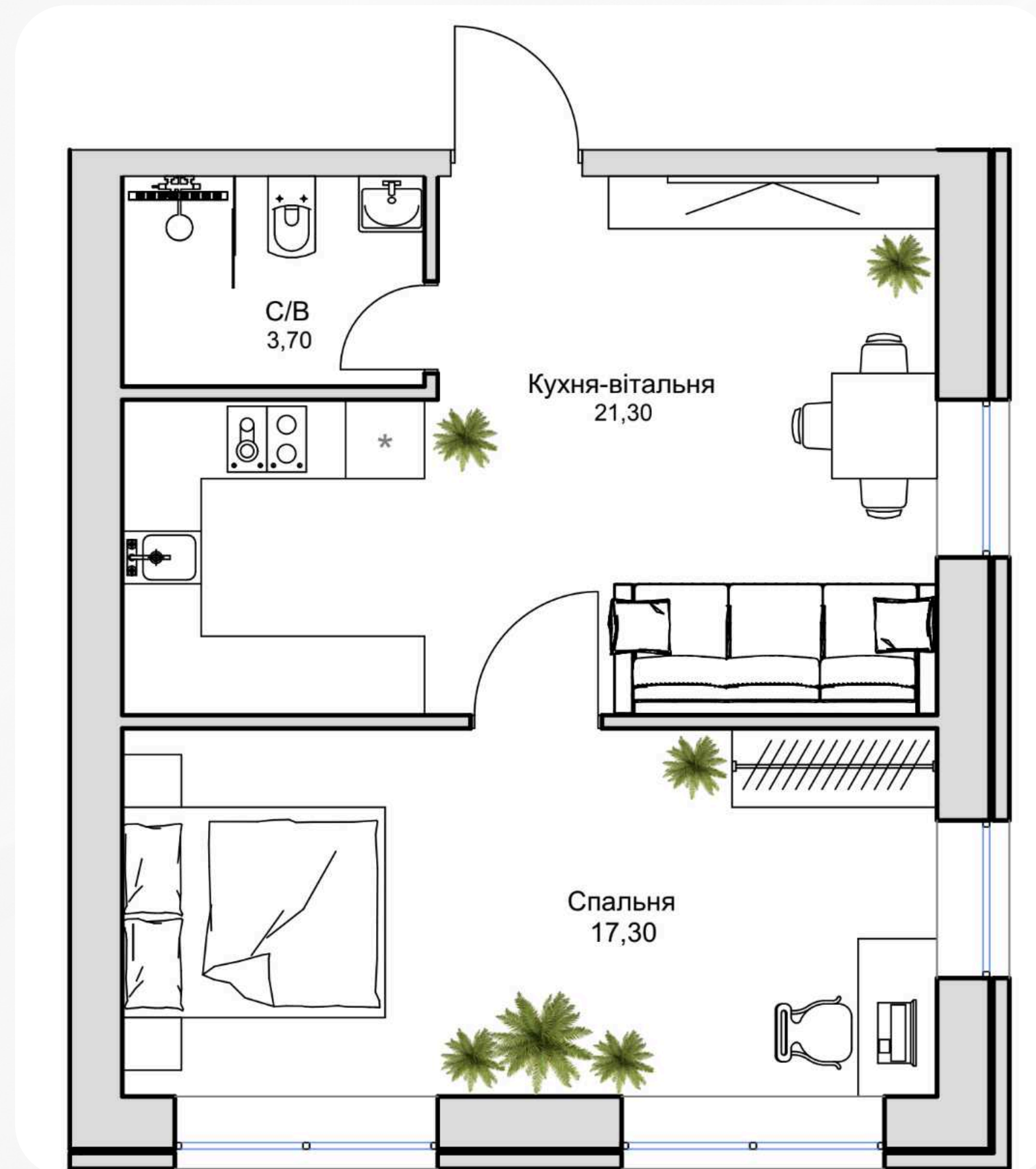
Однокімнатна 42 кв. м.
